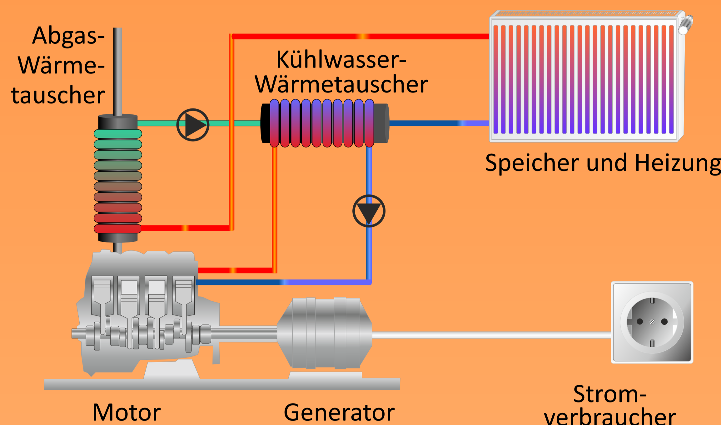
* Mini-BHKW (Blockheizkraftwerk)
